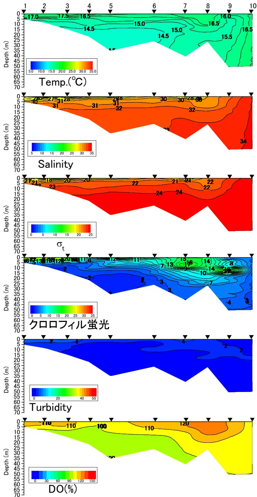
有明海中央ラインの水温(°C)、塩分、密度( \sigma_t )、クロロフィル蛍光強度、濁度、溶存酸素飽和度(DO%)の鉛直面図(国土交通省の調査による) (2017年4月20日)
